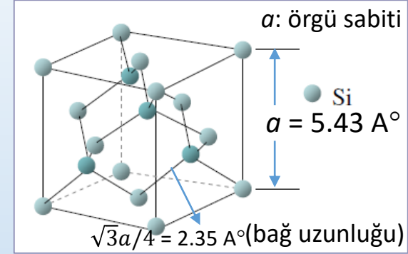
Silikon kristal birim hücresi (elmas yapı)
